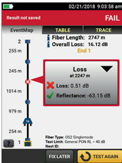
Link mit einem APC-Stecker, der als Dämpfungereignis angezeigt wird.
